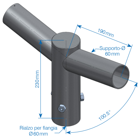
Flangia di montaggio a palo, supporto a 2 bracci Rialzo per flangia Ø60mm N° art. 135699 Rialzo per Ø76 mm N° art. 138136
