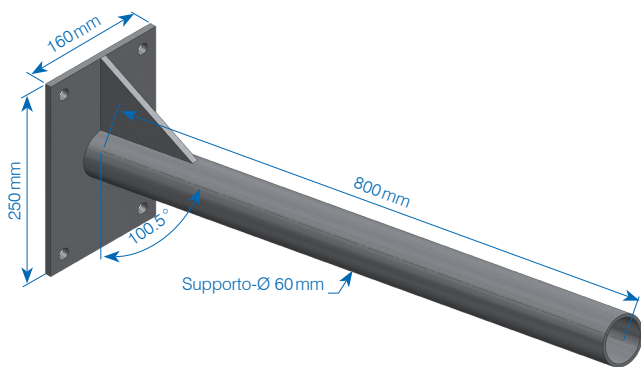
Supporto a muro N° art. 136695
