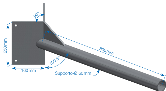
Supporto angolare N° art. 137688
