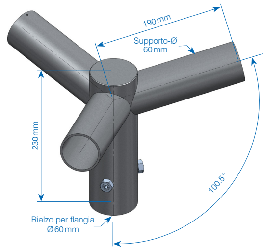
Flangia di montaggio a palo, supporto a 3 bracci Rialzo per flangia Ø60mm N° art. 135700 Rialzo per Ø76 mm N° art. 138137
