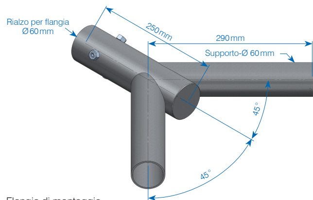
Flangia di montaggio N° art. 137727
